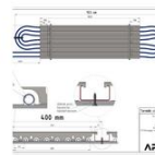
APPARAT rendszerlemez-es mennyezetfűtés+hűtés panelok
